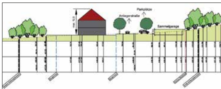
Erweiterungsteil Baugebiet „Altes Forsthaus“: Geländeschnitt mit der geplanten Sammelgarage
